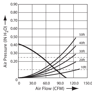
Fan Curve
