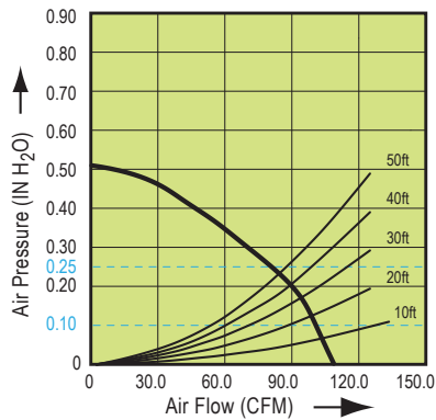
GBR100LED-DECOR Fan Curve
