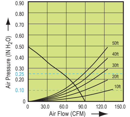
RAD80-DGL Fan Curve
