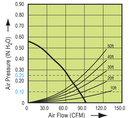
ITG100RLED Fan Curve
