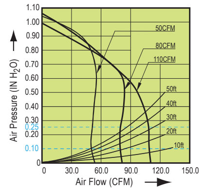
SLM50-110-C Fan Curve
