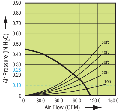
GBR100LED-DECOR Fan Curve
